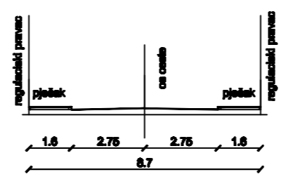
KARAKTERISTIČAN POPREČNI PRESJEK A - A M 1:200
