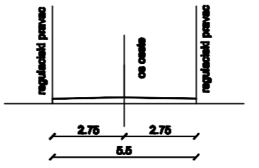
KARAKTERISTIČAN POPREČNI PRESJEK C - C M 1:200
